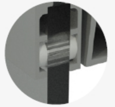
Cam Pim Detayı Glass Pin Feature
