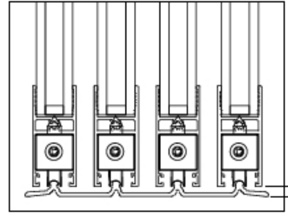
4'lü Eşiksiz Ray Sistemi Quadruple Non-lifted Rail System
